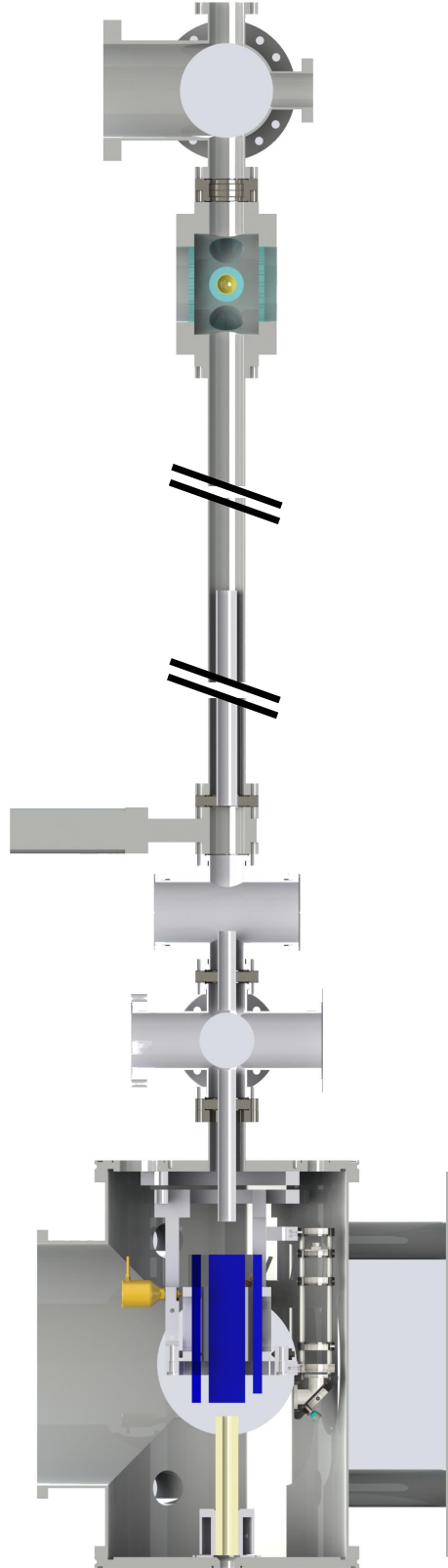
Abbildung 2.3: Oben: Schematische Zeichnung mit den wichtigsten Komponenten des experimentellen Aufbaus (nicht maßstabgetreu). Für eine Beschreibung der Komponenten siehe Text. Unten: Maßstabgetreue Konstruktionszeichnung, der ZSL wurde an den markierten Stellen in der Zeichnung gekürzt.
